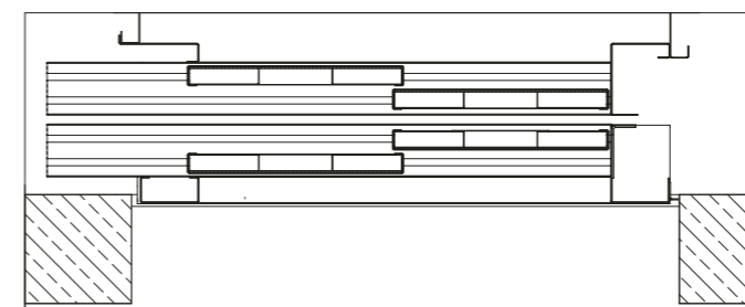
Horizontální řez kabinové a šachetní dveře s dveřní zárubní / napojení na zeď T1.
