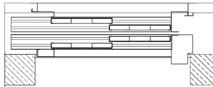
Horizontální řez jednostrannými dveřmi a servisní zárubní
